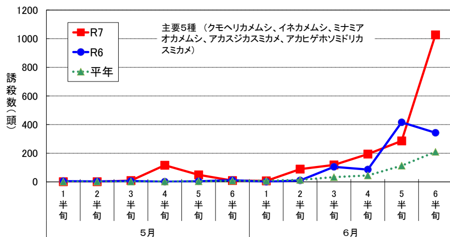
図 予察灯における斑点米カメムシ類主要5種の誘殺数 (県内3か所合計)
